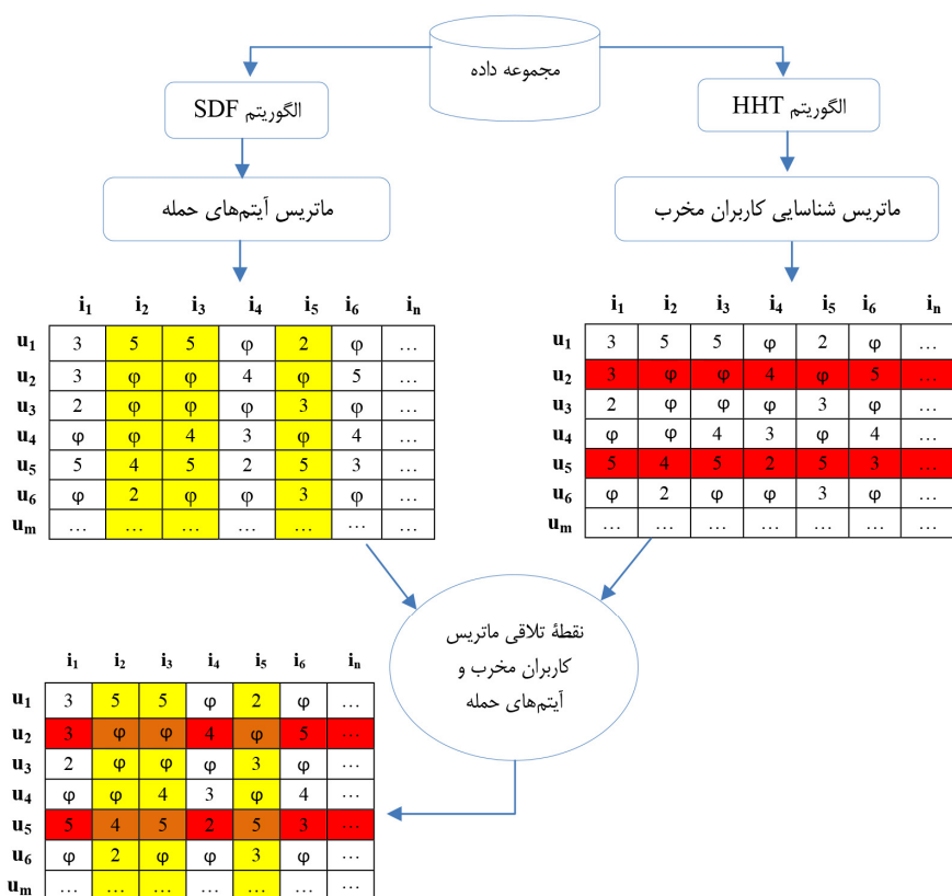
شکل ۱. معماری الگوریتم پیشنهادی
