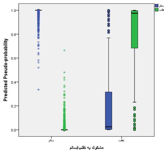
شکل ۳. نمودار پیش‌بینی - واقعی برای شبکه‌ی عصبی پرسپترون چندلایه مشکوک به تقلب/سالم
